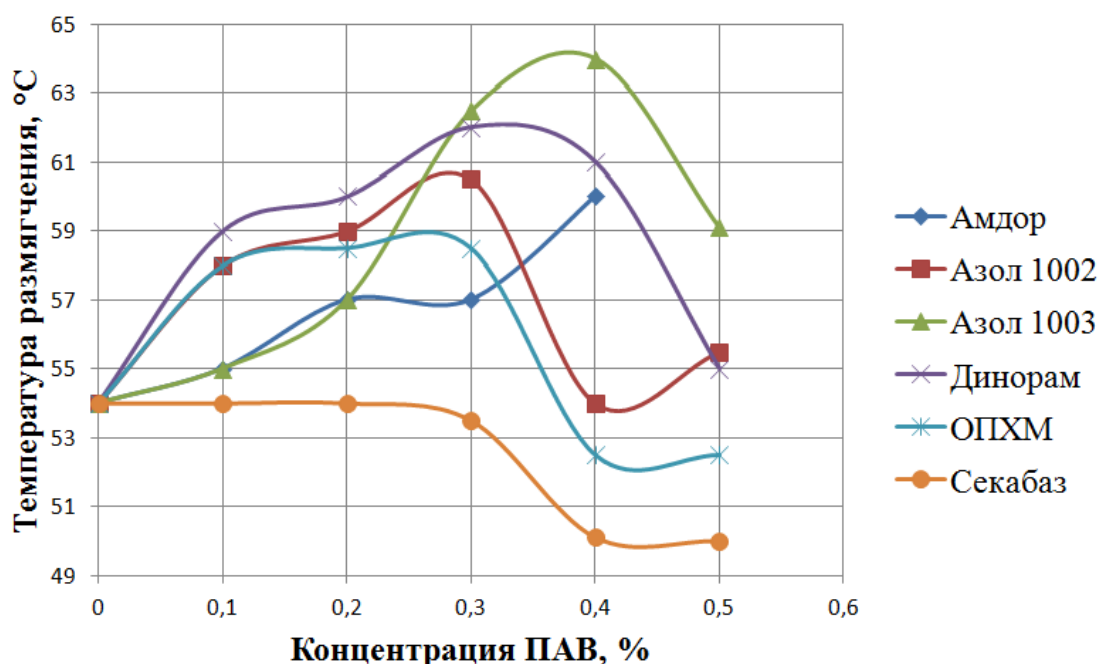
Рисунок 1 - Зависимость температуры размягчения битумполимерных вяжущих от концентрации ПАВ.
