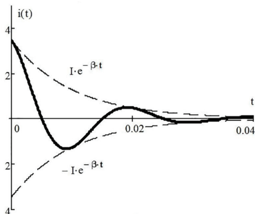
Рис. 1. Прерывание электроснабжения одного из потребителей в ЭТС с РГ
