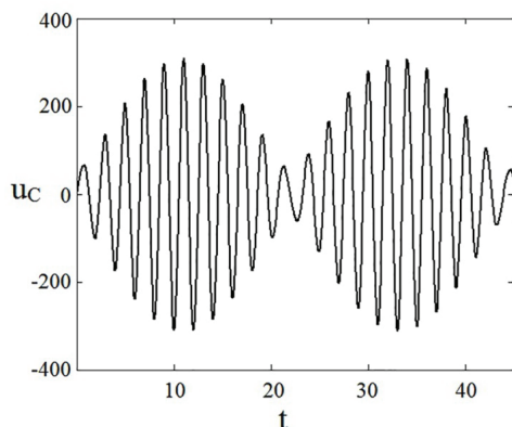
Рис. 5. Квазипериодические колебания напряжения на емкости
