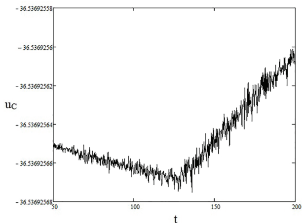
Рис. 7. Потеря устойчивости хаотического режима работы системы
