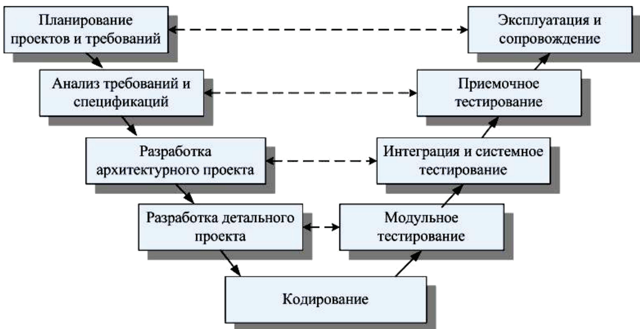
Рис. 9. Основные этапы процесса разработки ПО
