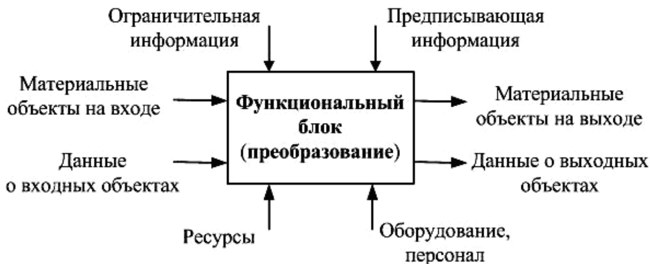
Рис. 12. Функциональный блок модели IDEF0
